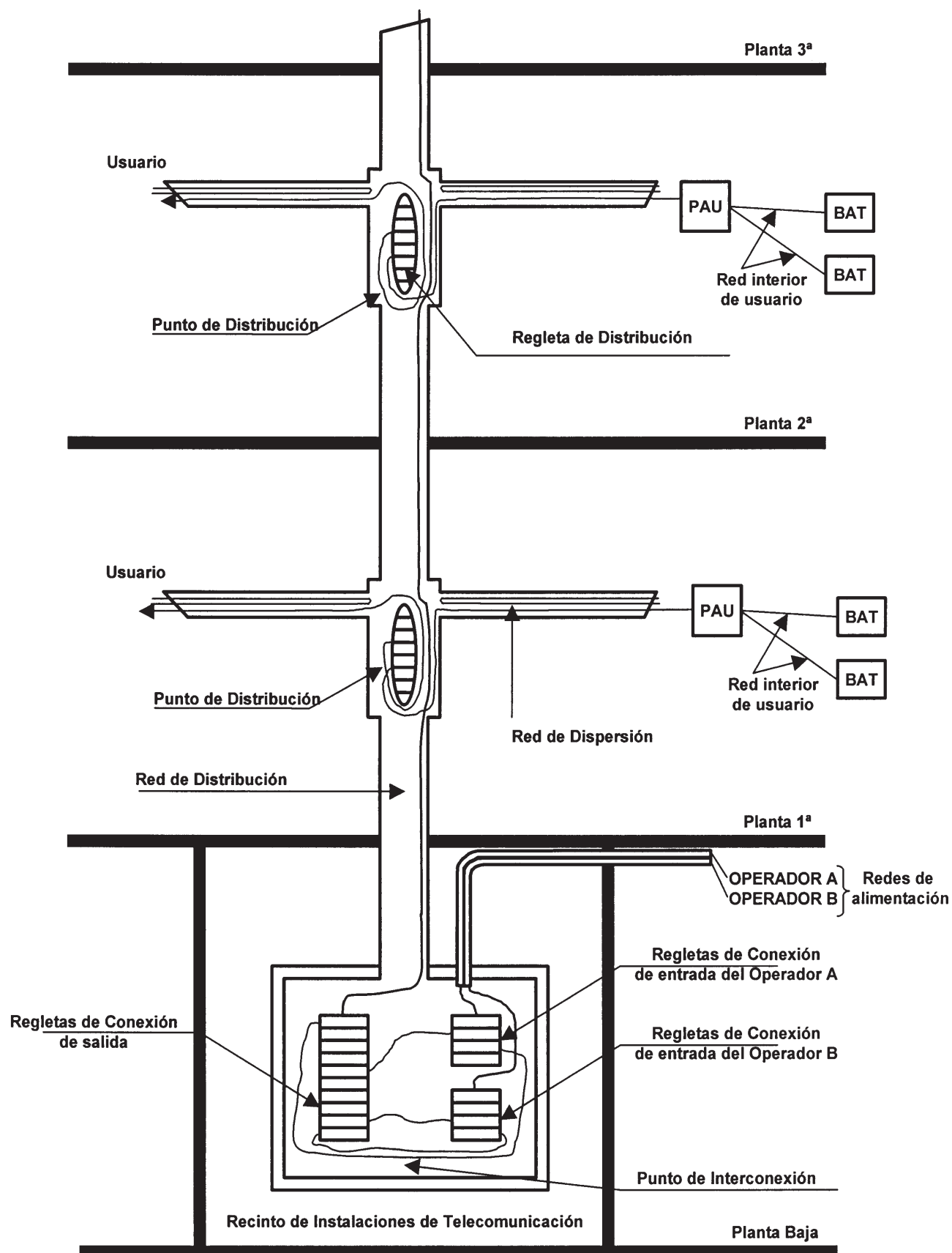
APÉNDICE 2 - ESQUEMA GENERAL DE RED
