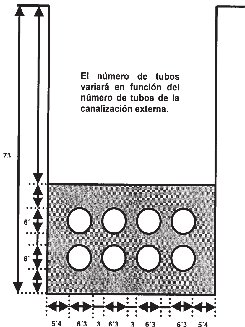
APÉNDICE 4: EJEMPLO DE SECCIÓN TRANSVERSAL DE CANALIZACIÓN DE ENLACE SUBTERRÁNEA DE 8 TUBOS.
